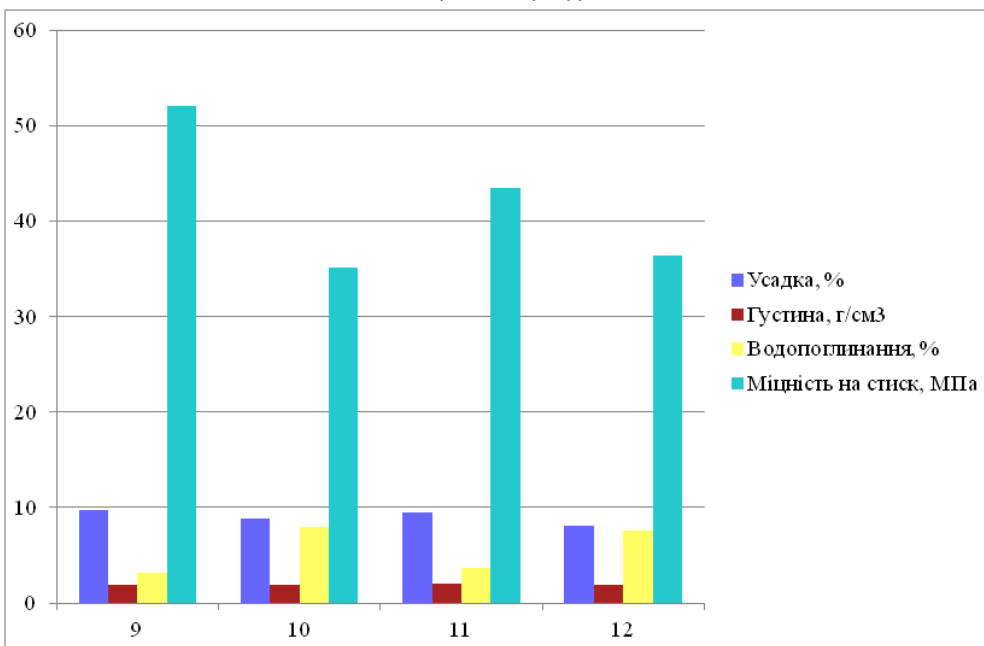
Рис. 2. Властивості кристалізаційної структури дослідних мас, отриманих в результаті математичного планування, випалених при температурі 1100 °C
