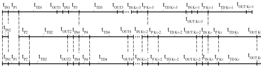
Рис. 1. Циклограма роботи доїльної установки з паралельно-прохідними станками
