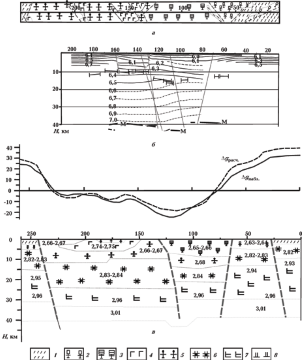
Рис. 4. Профиль ГСЗ XXIV. Геологическая обстановка (а), скоростной разрез (б), результаты сейсмогравитационного моделирования и модель распределения пород в земной коре (в): 1 — гнейсовые комплексы ингуло-ингулецкой серии, 2 — гранитоиды кировоградского комплекса, 3 — граниты новоукраинские, 4 — габбро-анортозиты, 5 — габбро-анортозиты, 6 — эндербиты, 7 — основные гранулиты, 8 — гнейсы пироксенового состава.
