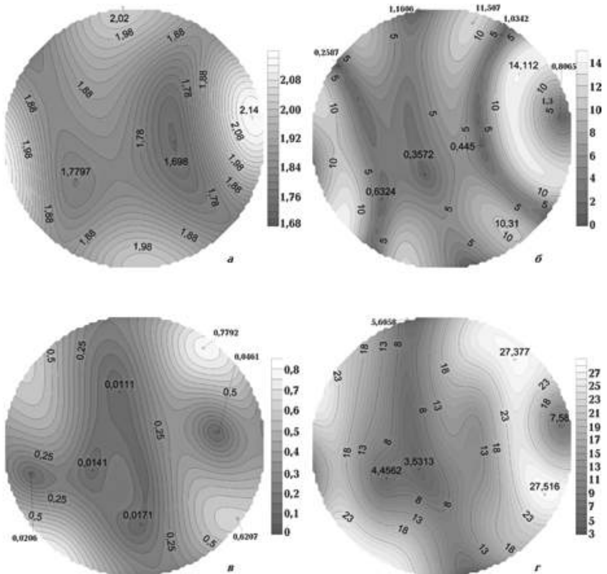
Рис. 7. Стереопроєкції розподілу величин для нахиленої глинистої товщі: a — індикатриси квазіпоздовжньої хвилі, ізолінії в км/с; b — кутів відхилення вектора пружних зміщень квазіпоздовжньої хвилі від хвильової нормалі, ізолінії в градусах; c — різниці між фазовими швидкостями поширення "швидкої" та "повільної" квазіпоперечних хвиль, ізолінії в км/с; d — диференціального коефіцієнта пружної анізотропії, ізолінії в %.
