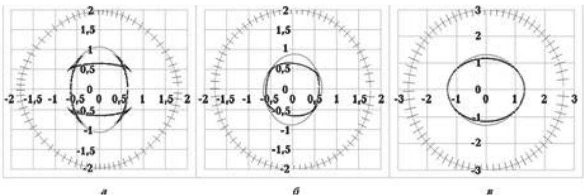
Рис. 12. Проекція хвильової поверхні квазіпоздовжньої P , "повільної" SV та "швидкої" SH квазіпоперечних хвиль на координатну площину X_1 X_3 (Polarization — напрямок поляризації). Умовні позначення див. на рис. 11.
