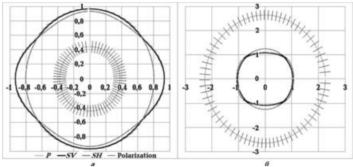
Рис. 13. Переріз поверхонь плавності (а) та рефракції (б) квазіпоздовжньої P , "повільної" SV та "швидкої" SH квазіпоперечних хвиль координатною площиною X_1 X_3 глинистого сланцю Пьєро на глибині 228,6 м (Polarization — напрямок поляризації).
