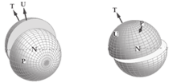
Рис. 15. Варіанти можливих розломів для землетрусу 06.01.2012.
