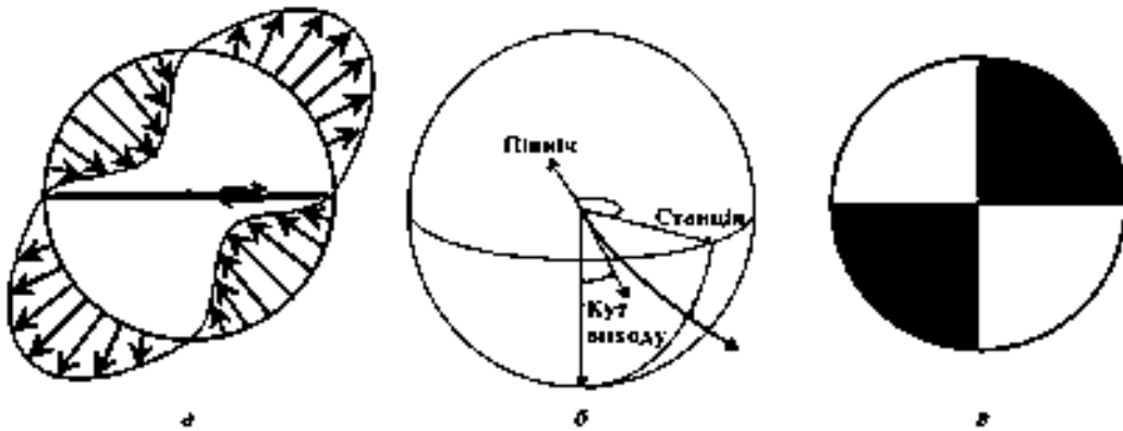
Рис. 1. Квадрантний розподіл даних сейсмічних станцій: a — діаграма випромінювання зсувної дислокації для P -хвиль; б — фокальна сфера; в — зображення механізму вогнища за допомогою стереографічної проекції.
