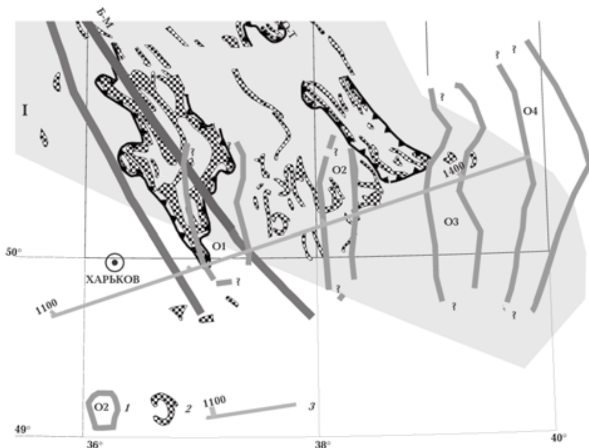
Рис. 4. Основные тектонические структуры ВКМ и объекты пониженного сопротивления (1), железистые кварциты (2) и положение геотраверса «Гранит» (3). Остальные обозначения см. на рис. 1.
