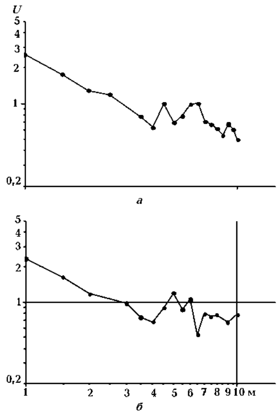
Рис. 6. График зависимости величины электромагнитного сигнала от глубины зондирования в билогарифмических координатах на частоте 2 МГц (а), 4 МГц (б).
