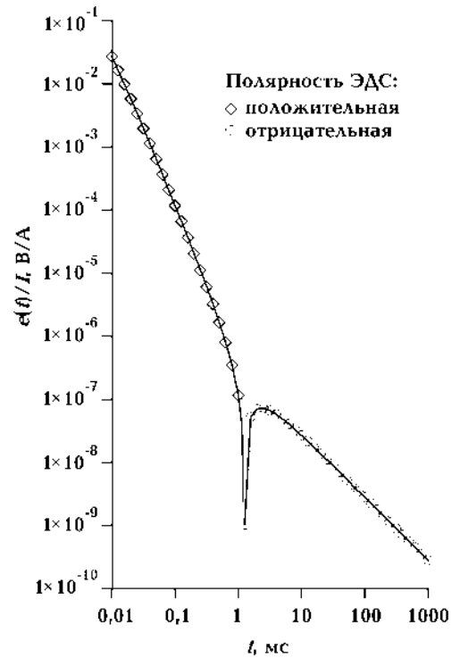
Рис. 2. Переходная характеристика установки с разнесенными петлями, расположенными на поверхности однородного полупространства ( \rho = 10^3 Ом·м, \kappa_0 = 0,001 ед. СИ). Параметры установки: размеры генераторной петли 100 \times 100 м, приемной петли — 50 \times 50 м, разнос — 80 м.
