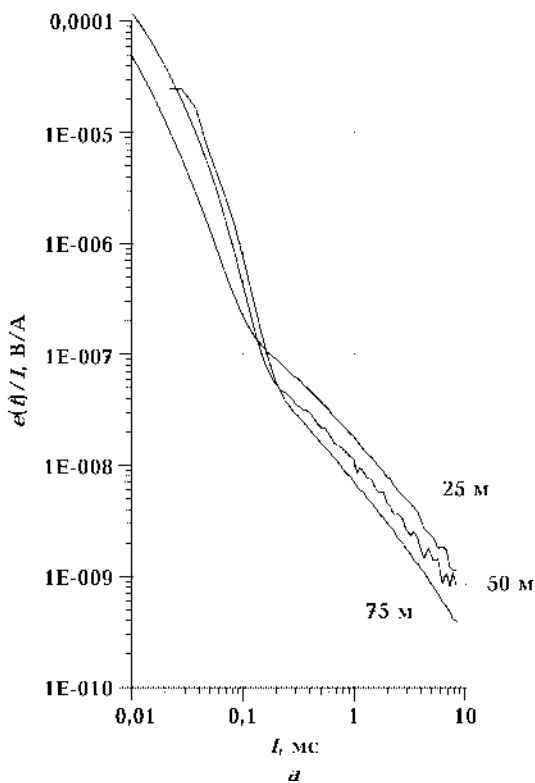
Рис. 5. Ручная инверсия параметрического зондирования: переходные характеристики, измеренные приемной рамкой, которая располагалась в центре квадратной генераторной петли с длиной стороны 25, 50 и 75 м (а); экспериментальный и модельный графики зависимости ЭДС на времени t=1 мс от длины стороны генераторной петли (б); модель среды (в). Значения ЭДС на рис. а, б приведены к рамке площадью 1 \text{ м}^2 .
