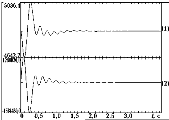
Рис. 14. Передаточные функции ЦР (трасса 1 — УК4, трасса 2 — УК13).
