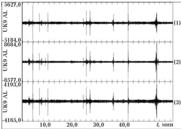
Рис. 8. Общий вид записей микросейсм, сделанных ЦР UK9 3 января 2007 г. с 01 ч 02 мин 21 с по 02 ч 01 мин 20 с. Каналы E, N, Z — трассы 1, 2, 3 соответственно.
