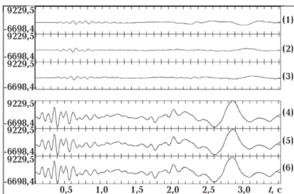
Рис. 3. Записи взрыва 29.12.2006 г. с/ст «СУМ» (ЦРИК9). Трассы 1—3 (датчик СМ3) и 4—6 (датчик ВЭГИК) в едином масштабе по оси Y.
