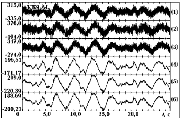
Рис. 9. Нефильтрованный (трассы 1, 2, 3) и фильтрованный (трассы 4, 5, 6) короткий участок микросейсм (27 с), представленных на рис. 8. Не содержит транспортную помеху.
