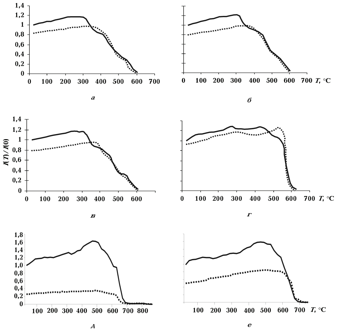
Рис. 2. Терромагнитный анализ образцов магнитного песка: а—в — Грузия (а — необогащенный, б — обогащенный, в — хвосты после обогащения); г—и — Крым (г — Партенит, д — Рыбачье, е — Новый Свет, ж — Николаевка, 2 км южнее пансионата, з — Николаевка, напро-
