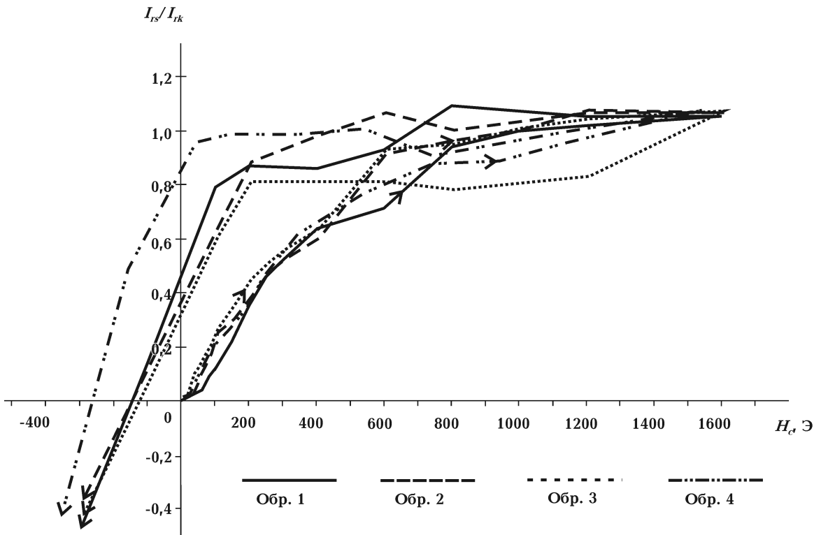
Рис. 3. Результаты определения коэрцитивной силы ( H_c ) исследуемых образцов.
