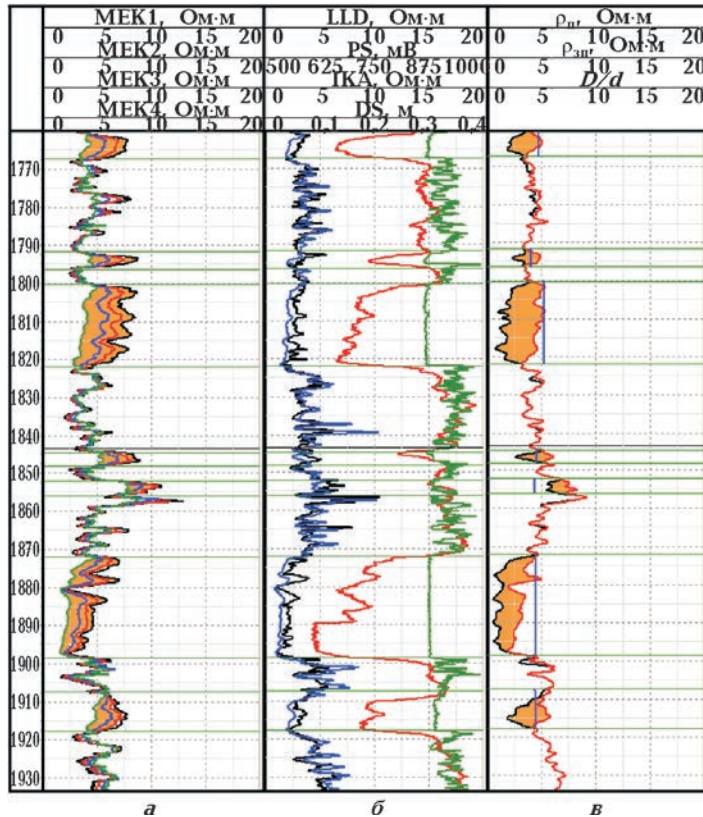
Рис. 5. Интервал скважины (Днепроовско-Донецкая впадина, Веселовское месторождение, у. э. с. скважины 0,3 \text{ Ом} \cdot \text{м} ): а — кривые зондов “псевдо-бокового” каротажа, синтезированные по данным 14-ти зондов МЭК-М; б — у. э. с. (LLD — бокового каротажа БК-3; ИКА — индукционного каротажа 6Ф1); PS — кривая потенциала самопроизвольной поляризации; DS — диаметр скважины; в — рассчитанные по данным МЭК-М у. э. с. пласта и зоны проникновения, D/d — рассчитанное по данным МЭК-М отношение диаметра зоны проникновения к номинальному диаметру скважины.
