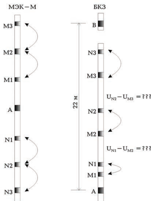
Рис. 2. Геометрия аппаратуры МЭК-М и БКЗ. Различие в измерении разности потенциалов между измерительными электродами.
