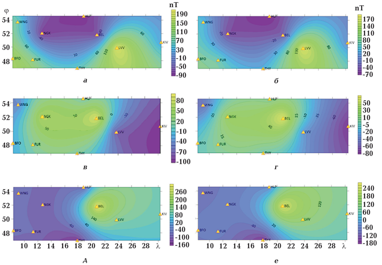
Рис. 5. Карти величин \Delta B_x (а), \Delta B_y (б), \Delta B_z (А) і їх модельних значень \Delta B_{xm} (б), \Delta B_{ym} (г), \Delta B_{zm} (е).
