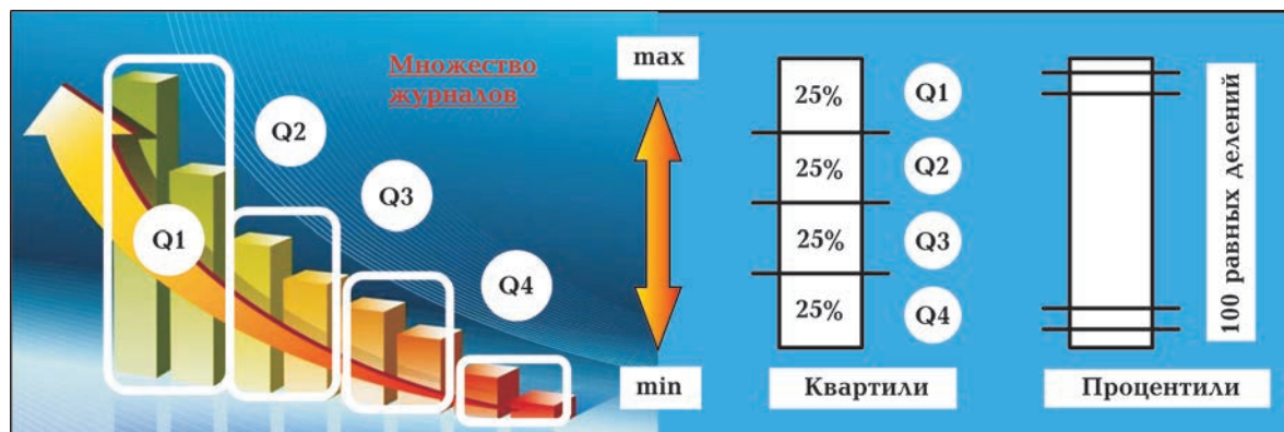
Рис. 6. Квартили и процентиля.
