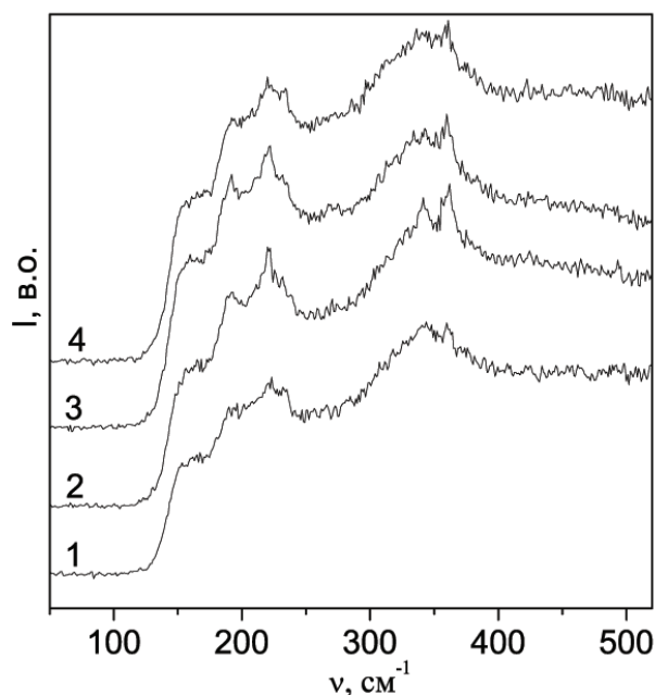
Рис. 6: Раманівські спектри свіжоприготованих плівок As_{40-x}Sb_xS_{60} . x , ат. %: 1–1.6; 2–4; 3–6; 4–8.
