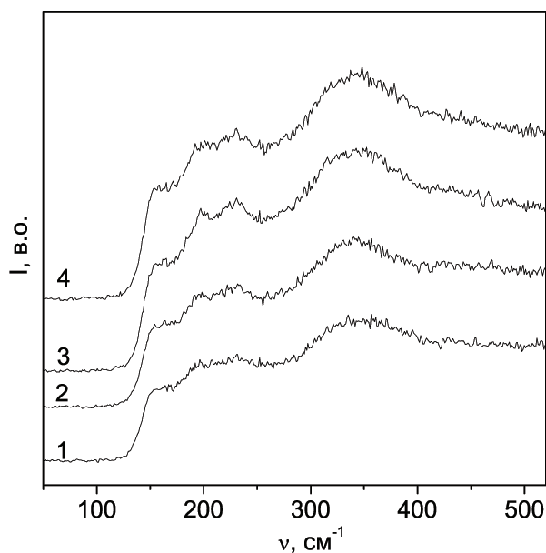
Рис. 7: Раманівські спектри опромінених протягом 2 хв. плівок As_{40-x}Sb_xS_{60} . x , ат. %: 1–1.6; 2–4; 3–6; 4–8.
