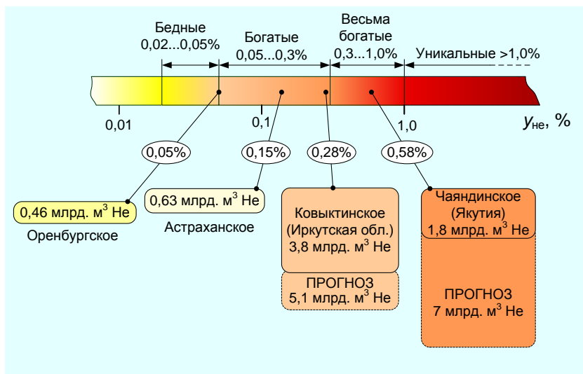
Рисунок 1. Градація месторождений природного газа по содержанию гелия. (Для наглядности показаны объемы и средние концентрации He в некоторых газогелиевых провинциях России)
