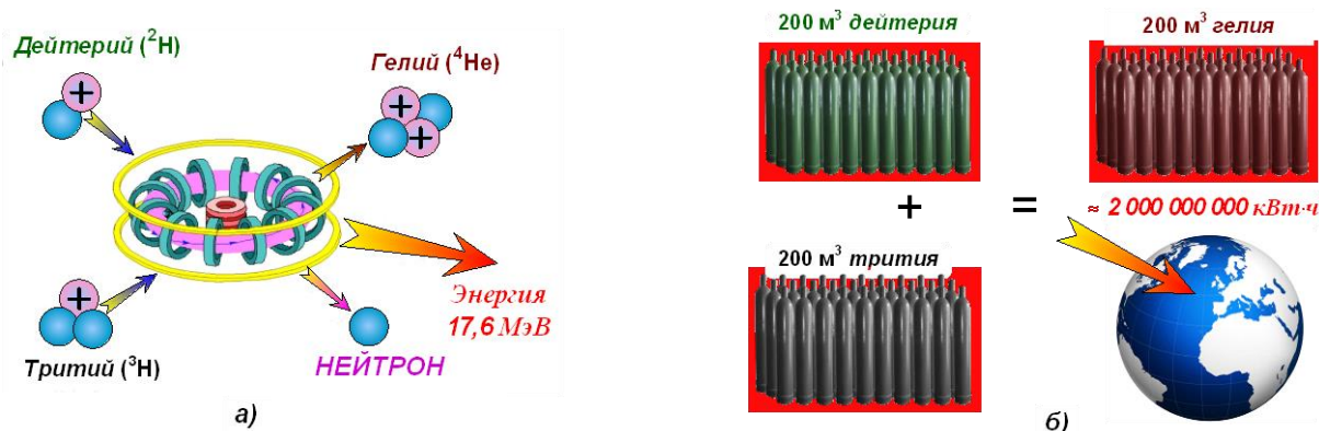
Рисунок 4. Один из типов термоядерной реакции, сопровождаемой получением изотопа ^4\text{He} ; а) - на уровне элементарных частиц; б) – на макроуровне (1 час работы электростанции с кпд 50%, обеспечивающей глобальные потребности человечества)
