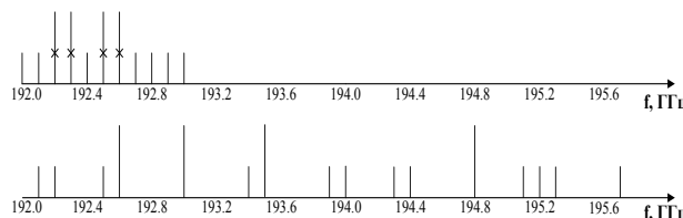
Рис. 2. Сравнение методов назначения длин волн на ребре между 1 и 2 вершиной
