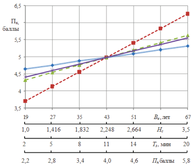
Рис. 1. Характеристический график изменения функционального состояния водителя в транспортном заторе: — P_n ; — T_z ; — H_c ; — V_v
