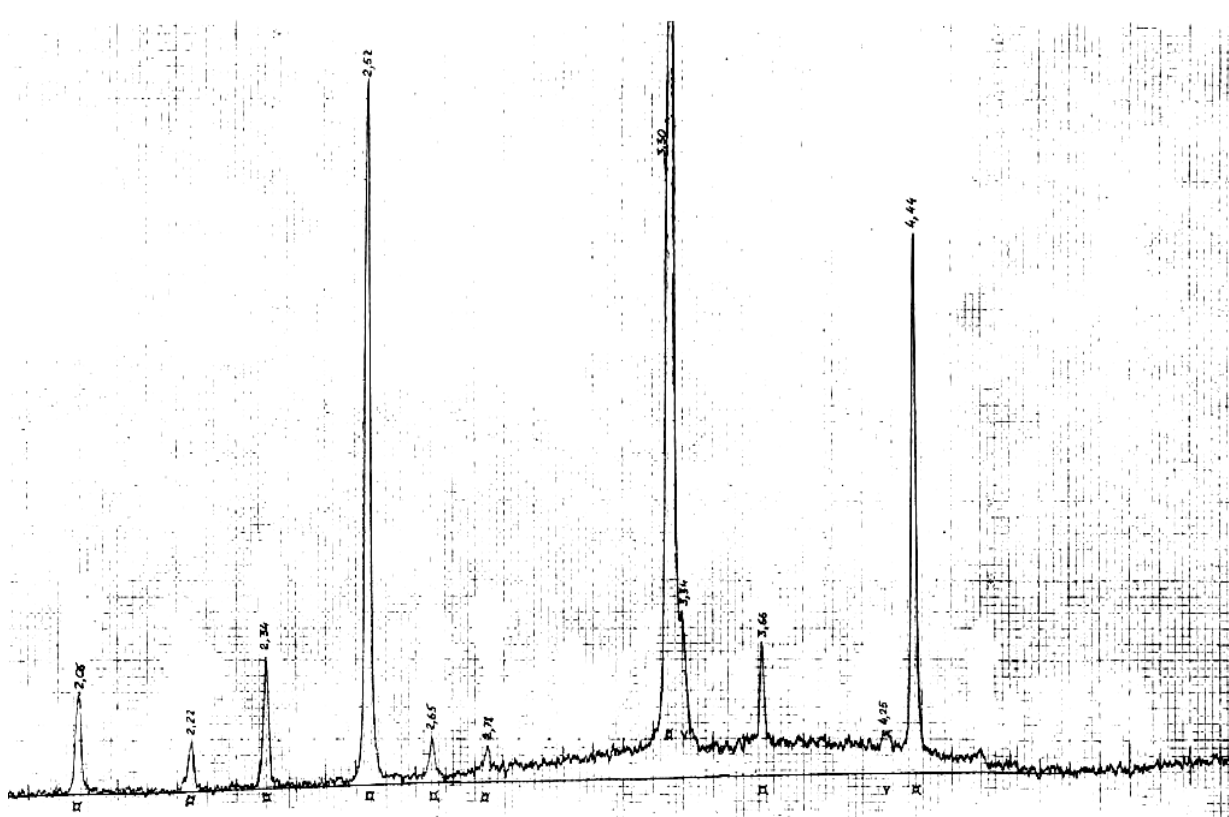
Рис. 5. Дифрактограма глазурі Н 07 після випалу на 1220°С .Позначення: □ циркон, v кварц
