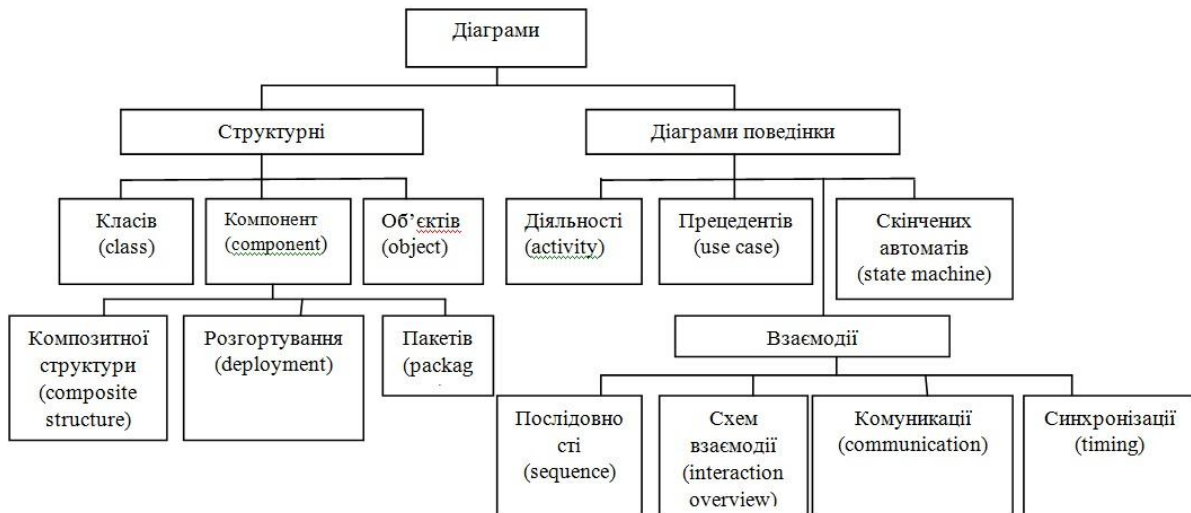
Рис. 1. Типи діаграм UML
