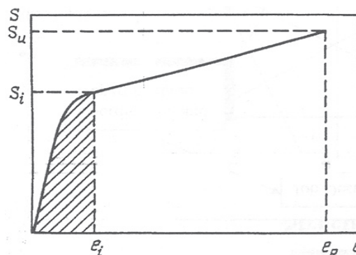
Рис. 1. Схема определения текущих значений поврежденности при ползучести
