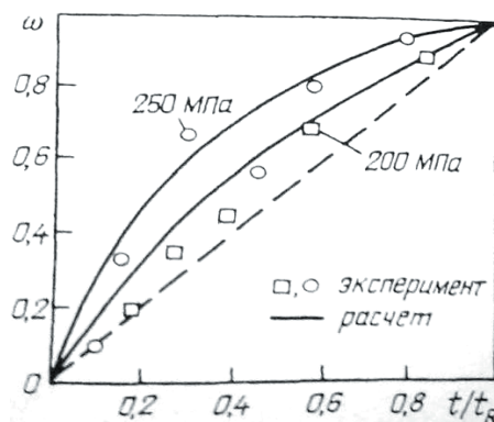
Рис. 3. Кинетические кривые поврежденности образцов сплава ХН55МВЦ при температуре \theta = 650^\circ\text{C}
