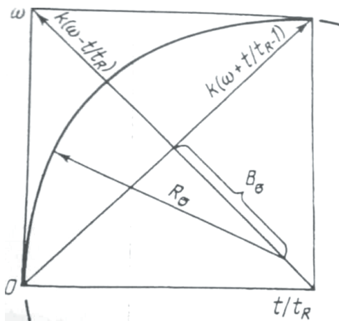
Рис. 2. Схема аппроксимации кинетической кривой поврежденности
