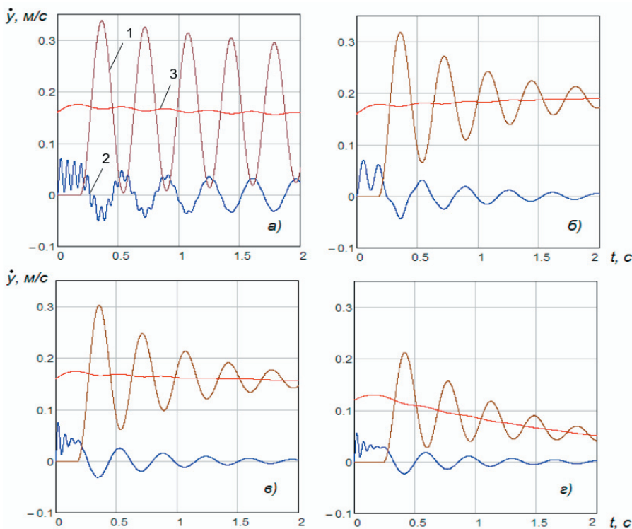
Рис. 3. Графік швидкостей при різних робочих характеристиках гасителя коливань: а – без гасителя коливань; б – лінійна характеристика; в – прогресивна характеристика; г – регресивна характеристика; 1- швидкість зведеної маси вантажу ( \dot{y}_n ); 2 – швидкість зведеної маси стріли ( \dot{y}_c ); 3 – швидкість зведеної маси приводу ( \dot{y}_d )
