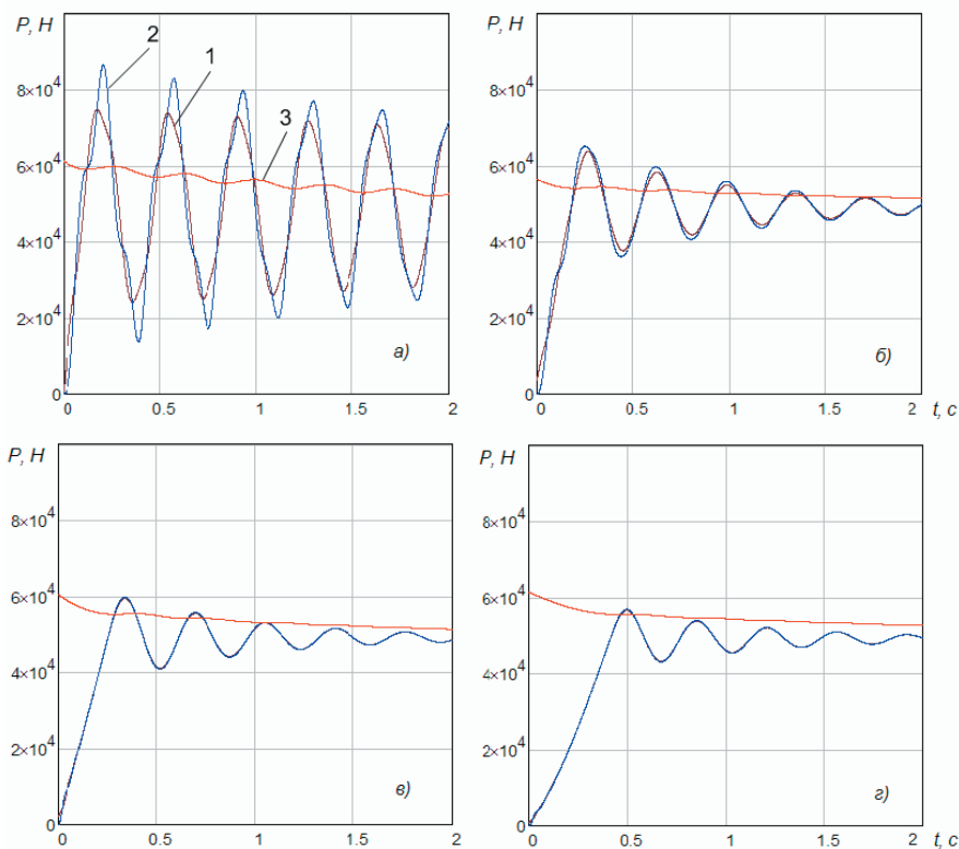
Рис. 2. Графіки зміни зусиль в часі при різних робочих характеристиках гасителя коливань: а – без гасителя; б – лінійна характеристика; в – прогресивна характеристика; г – регресивна характеристика; 1 – зусилля в вантажних канатах ( P_k ); 2 – зусилля в стрілі ( P_c ); 3 – зусилля приводу ( P_d )
