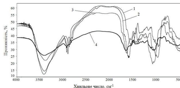
Рис. 1. Порівняння ІЧ-спектрів проникності у відношенні до хвильового числа кисломолочних напоїв «Фітолакта» (1), «Пряний» (2) та «Ароматний» (3) з ІЧ-спектром традиційного кефіру за ДСТУ 4417:2005 (4) як аналог
