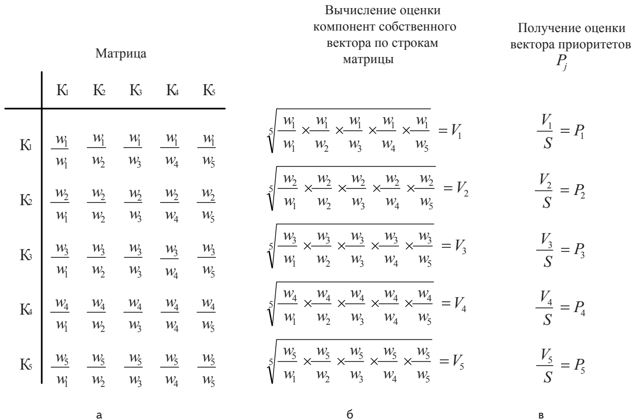
Рис. 2. Оценка вектора приоритетов: а – матрица, б – вычисление оценки компонент собственного вектора, в – получение оценки вектора приоритетов
