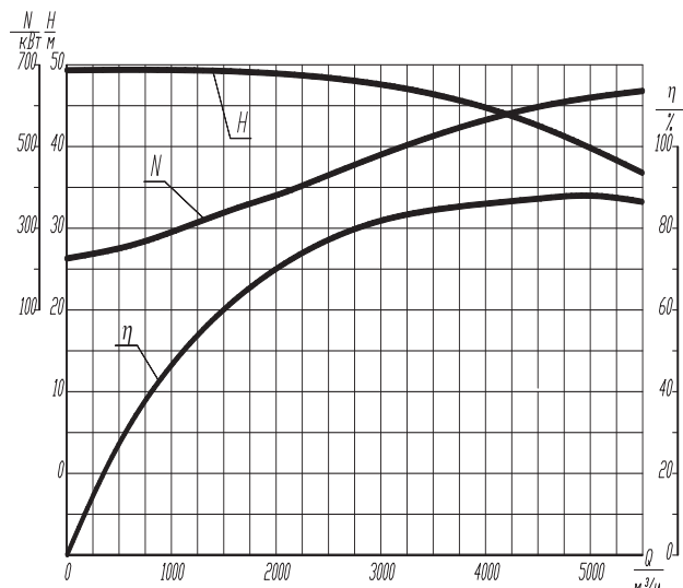
Рис. 2. Энергетические характеристики модернизированного насоса 24 НДС (с параметрами в рабочей точке Q = 5500 \text{ м}^3/\text{ч} , H = 38 \text{ м} )
