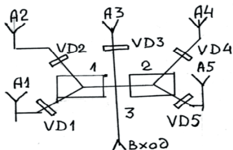
Рис. 1: а – структурная схема; б – общий вид конструкции антенного модуля
