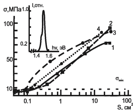
Рис. 1. Зависимость механических напряжений от площади поверхности кристаллов нелегированного GaAs, выращенных методом Чохральского. 1, 2 – кристаллы, полученные с избытком мышьяка; 3, 4 – с его недостатком. 1, 3 - N_d = (2-3) \cdot 10^4 \text{ см}^{-2} ; 2, 4 - N_d = (5-6) \cdot 10^5 \text{ см}^{-2}
