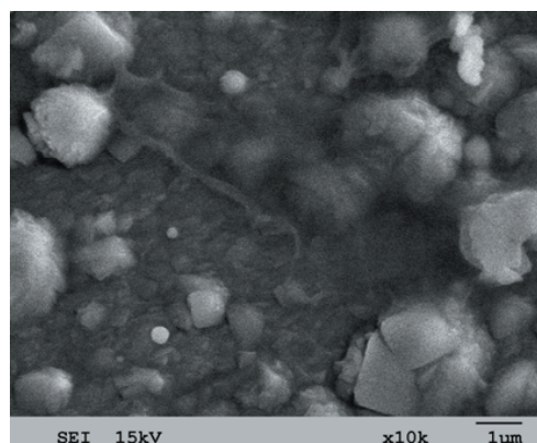
Рис. 2. Морфология поверхности покрытия, осажденного при потенциале подложки -5 В. U_{ни} = -2 кВ, I_d = 85 А, p_N = 0,66 Па, f = 7 кГц
