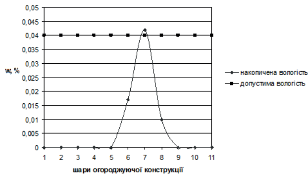
Рис. 1. Залежність розподілення вологи у шарах не утепленої зовнішньої огорожуючої конструкції для квітня, де 1, 2, 3...11 – шари цегляної кладки
