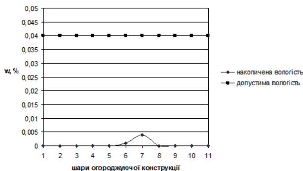
Рис. 4. Залежність розподілення вологості у шарах утепленої з обох боків зовнішньої стіни для березня, де 1 і 11 – шари утеплювача; 2, 3, 4...10 – шари цегляної кладки
