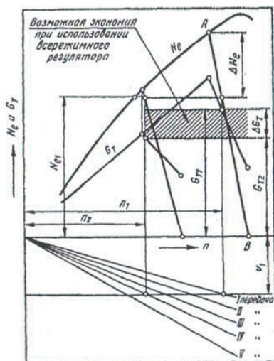
Рис. 1. Графічний аналіз впливу загально режимного регулятора на показники роботи двигуна за В.М. Болтинським
