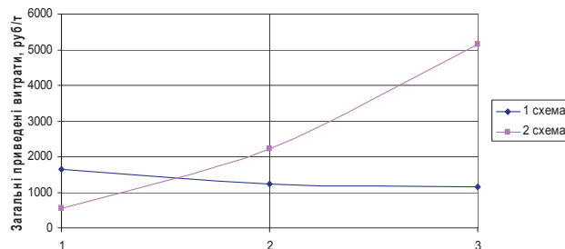
Рис. 4. Графік залежності загальних приведених витрат від мінімальних, середніх та максимальних значень вхідних параметрів для двох ТТС
