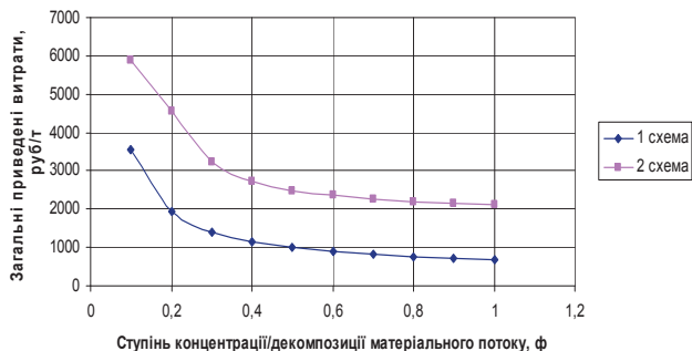
Рис. 3. Графік залежності загальних приведених витрат від ступеня концентрації/декомпозиції матеріального потоку для двох ТТС
