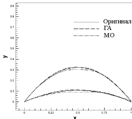
Рис. 5. Оригинальный и перепроектированный профиль лопатки
