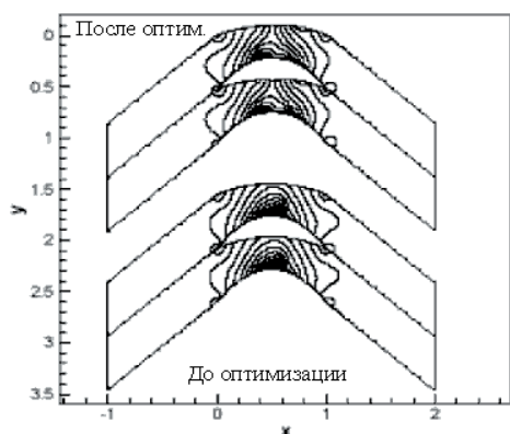
Рис. 3. Контурное распределение числа Маха для каскада компрессора с использованием алгоритма Модельного отжига
