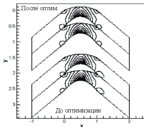
Рис. 1. Контурное распределение числа Маха для каскада компрессора с использованием ГА
