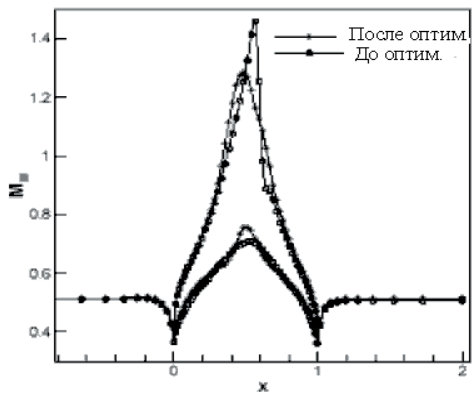
Рис. 2. Распределение числа Маха вдоль профиля для каскада компрессора с использованием ГА
