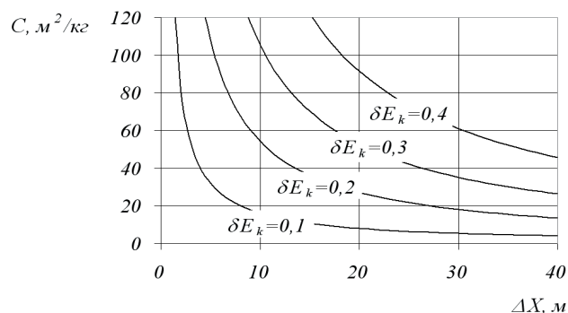
Рис. 2. Залежність балістичного коефіцієнту металюого елемента від діапазону відстаней застосування зброї
