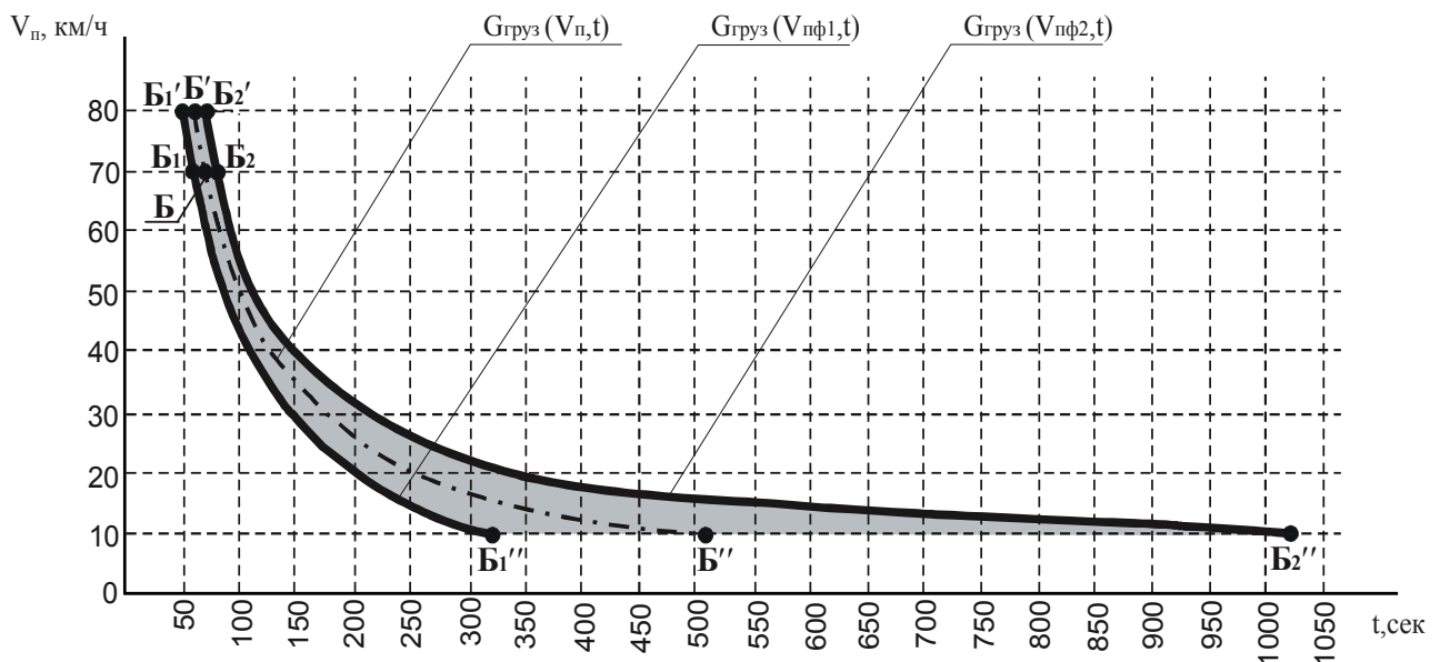
Рис. 2. Графики функций G(V_{п,t}) , G(V_{пф1,t}) и G(V_{пф2,t}) времени вступления грузовых поездов в опасную зону переезда при наличии погрешностей в определении скорости их движения
