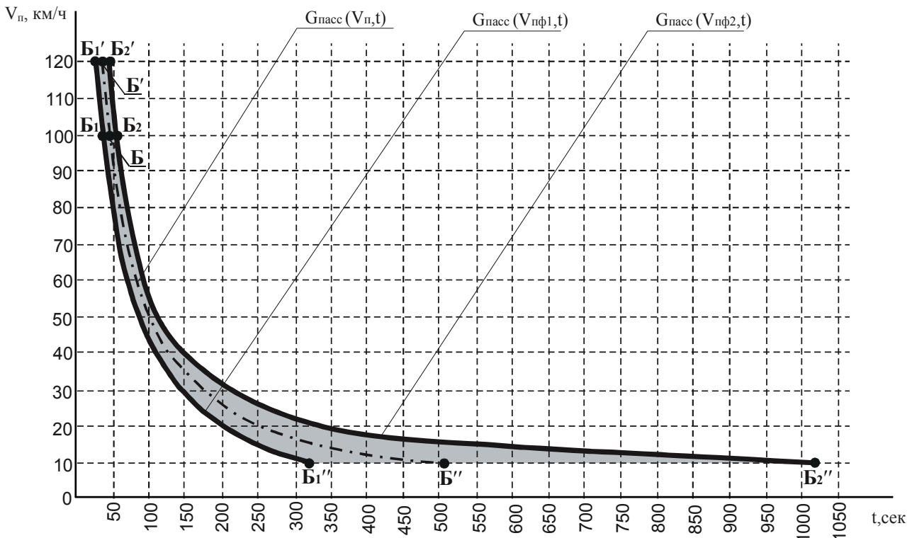
Рис. 3. Графики функций G(V_p, t) , G(V_{пф1}, t) и G(V_{пф2}, t) времени вступления пассажирских и пригородных поездов в опасную зону переезда при наличии погрешностей в определении скорости их движения
