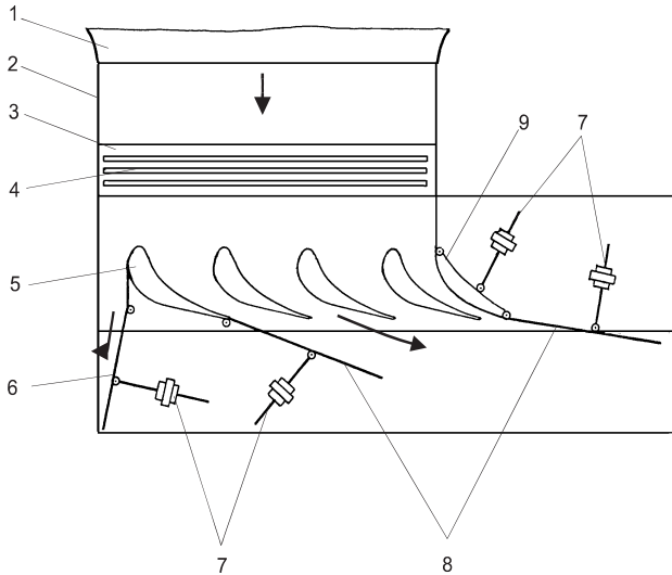
Рис. 2. Схема рабочей части экспериментальной установки: 1— сопло Витошинского; 2— ограничивающие стенки; 3— сменная пластина; 4— щели для слива пограничного слоя; 5— лопатки исследуемой решетки; 6— поворотная пластина канала; 7— винтовые пары; 8— регулировочные створки; 9— поворотная профилированная стенка
