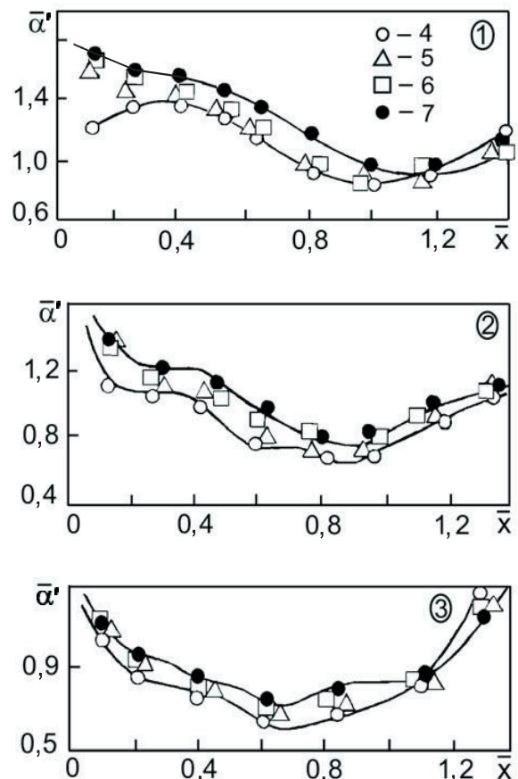
Рис. 4. Относительное изменение интенсивности локального теплообмена вдоль торцевой поверхности криволинейного канала ( Re_{\tau} = 3,7 \cdot 10^5 ; \delta_{вх} = 1\text{мм} ) по сравнению с плоской пластиной: 1...3 — около вогнутой стенки, средней линии и выпуклой стенки канала соответственно; 4...7- \bar{h} = 1,0 ; 0,47; 0,24 и 0,14 соответственно
