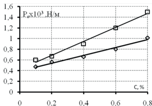
Рис. 2. Залежність ГНЗ МАШ від концентрації E472e системи «молоко-E472e» за температури 20 \pm 1 °C на межі розділу фаз: □ – вода-олія; ◇ – вода-повітря
