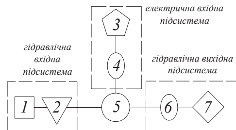
Рис. 2. Структурна схема комплексу подачі та розподілу води
