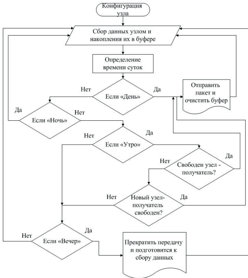
Рис. 3. Алгоритм управления передачей данных для узла БСС
