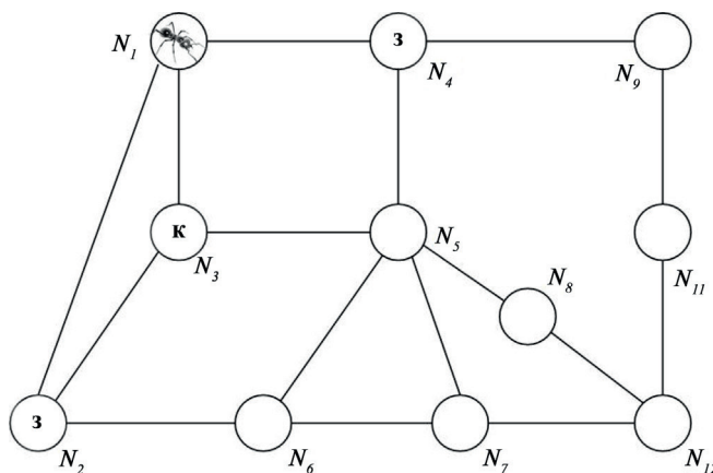
Рис. 4. Работа муравьиного алгоритма с применением семафоров
