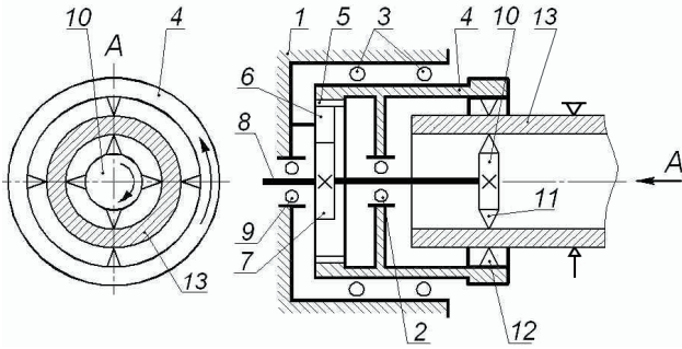
Рис. 3. Пристрій для одночасної обробки внутрішньої та зовнішньої поверхонь
