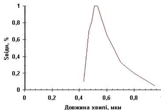
Рис. 1. Відносна спектральна характеристика S(λ) ФЕП
