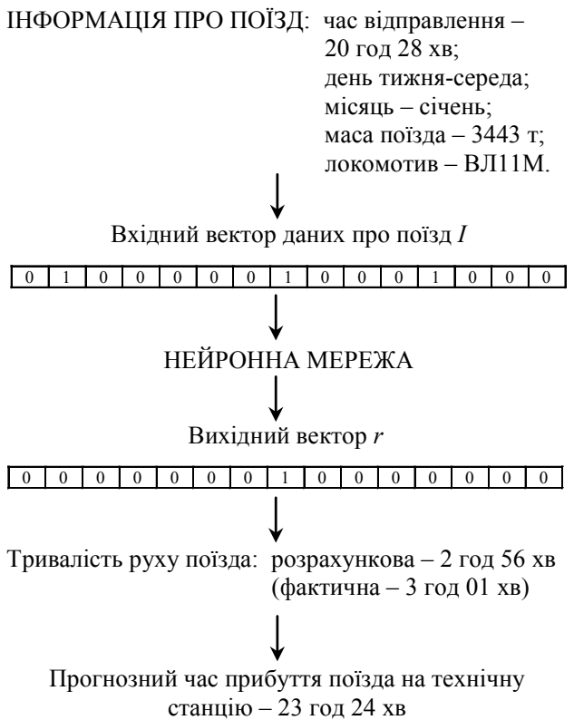
Рис. 3. Алгоритм роботи перцептрона
