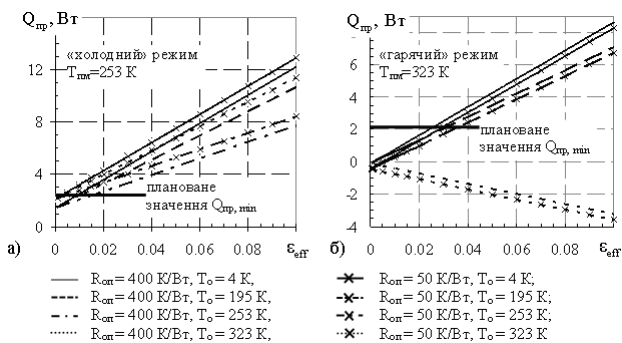
Рис. 2. Мінімальне значення тепловантаження приладу для початку функціонування пасивної СЗТР у «холодному» (а) та «гарячому» режимах. Дані отримано при Q_{ГРТТ,min} = 1 Вт, R_{каб} = 145 К/Вт
