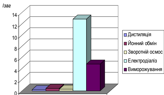
Рис. 4 - Порівняння способів опріснення за показником I_{zag} для виробництва пива
