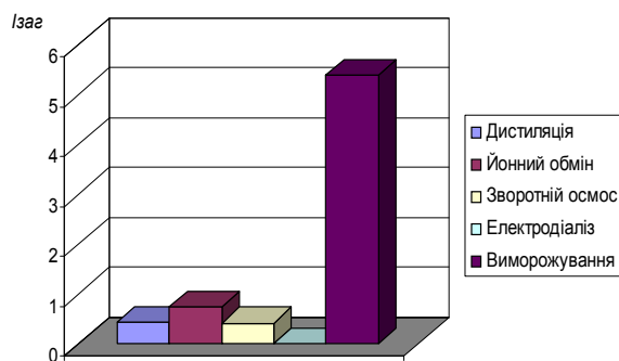
Рис. 5 - Порівняння способів опріснення за показником I_{zag} для виробництва безалкогольних напоїв
