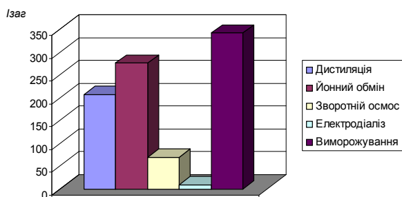
Рис. 3 - Порівняння способів опріснення за показником I_{zag} для виробництва горілки
