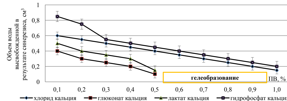
Рис. 3. Зависимость синергических свойств растворов ПВ от массовой доли пектина в растворе и природы солей кальция
