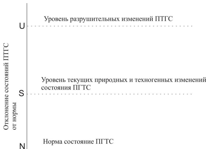
Рис.1. Основные уровни состояния геосистем: NS – степень отклонения состояния объекта от нормы; SU – степень приближения объекта к уровню разрушения его структуры (по В.А. Бокову, А.В. Лущику)
