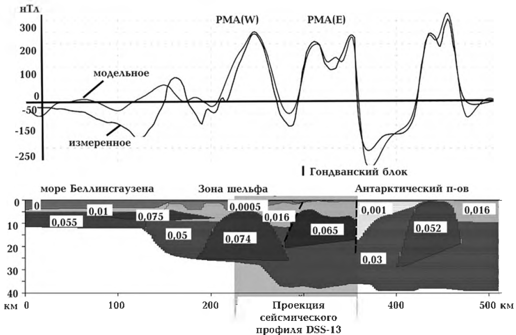
Рис. 5. Магнитная модель земной коры вдоль профиля III—III от моря Беллинсгаузена до Антарктического полуострова, по [Yegorova, Bakhmutov, 2013]. Числа — значения магнитной восприимчивости в ед. СИ. Положение профиля см. на рис. 1.
