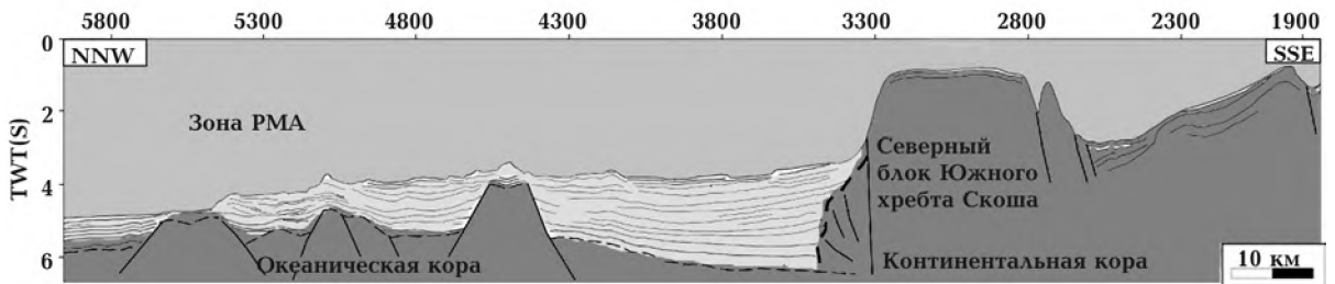
Рис. 10. Сейсмический профиль SA-500-002 через зону РМА (Е) и северный блок Южного хребта Скоша, по [Civile et al., 2012]. Положение профиля см. на рис. 1.
