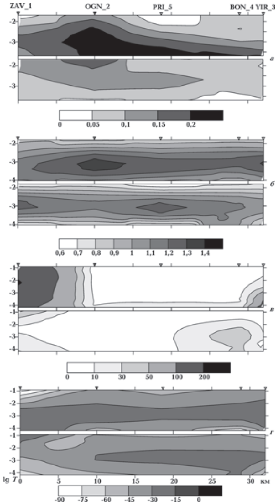
Рис. 10. Псевдорезрезы МТ/МВ параметров вдоль профиля Керчь-3: а–г — согласно условным обозначениям рис. 2.
