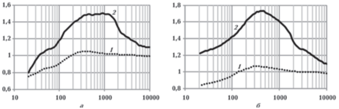
Рис. 7. Значения главных компонент M_{yy} (1) и M_{xx} (2) тензора горизонтального аномального поля в пункте SOL-6 при нормировке на данные пунктов VID-8 (а) и YUZ-7 (б).
