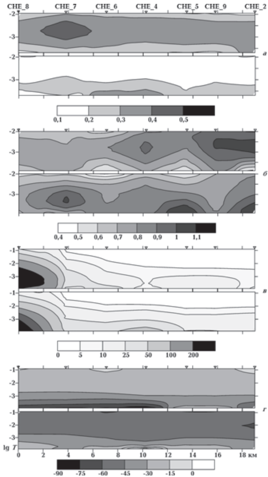
Рис. 2. Псевдоразрезы МТ/МВ параметров вдоль профиля Черноморский: a — значения компонент типперов \text{Re}W и \text{Im}W ; б — значения главных компонент M_{yy} и M_{xx} тензора горизонтального аномального поля; в — значения кажущегося сопротивления амплитудных кривых \rho_{xy} и \rho_{yx} ; г — фазовые \varphi_{xy} и \varphi_{yx} кривые импеданса. Вертикальная шкала — \lg T .
