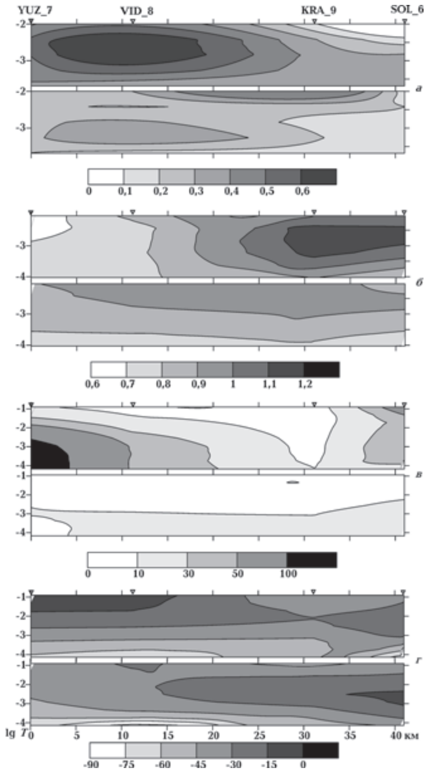
Рис. 6. Псевдоразрезы МТ/МВ параметров вдоль профиля Джанкойский: a—г — согласно условным обозначениям рис. 2.
