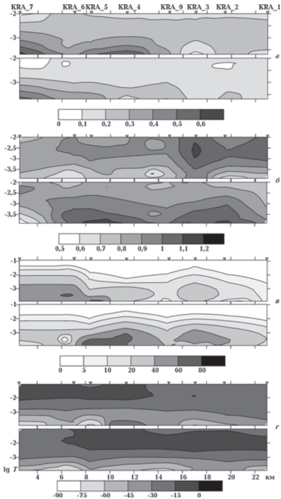
Рис. 3. Псевдоразрезы МТ/МВ параметров вдоль профиля Краснополянский: а—г — согласно условным обозначениям рис. 2.
