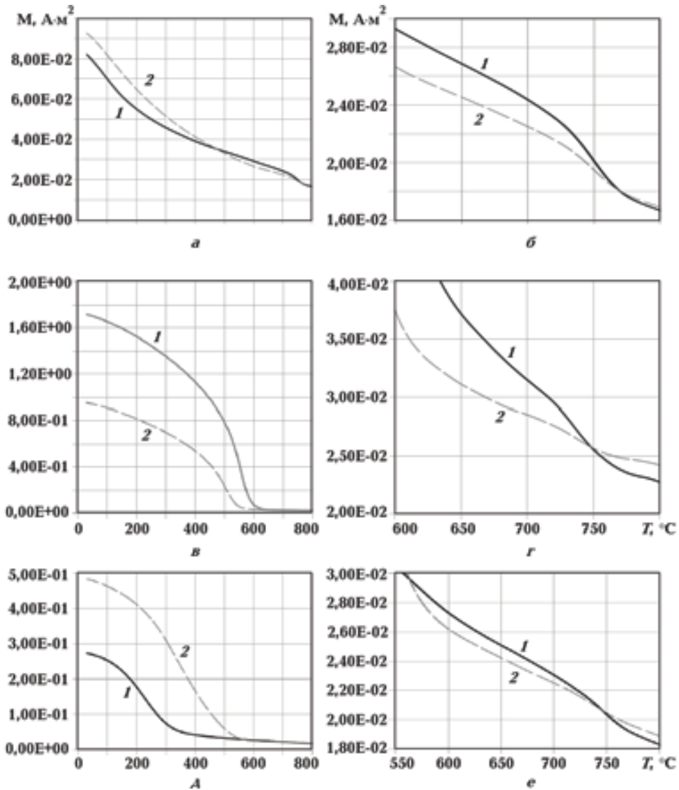
Рис. 1. Примеры результатов ТМА: 1 — первый нагрев, 2 — второй нагрев; а, б — обр. СВ-462, лерцолит, Приморье (кривая имеет форму гиперболы); зафиксировано железо с T_C = 770^\circ\text{C} ; в, г — образец А-10, лерцолит, Сирия (в — кривая M(T) Q-типа, г — зафиксировано железо с T_C = 765^\circ\text{C} ); д, е — обр. 2793-3, базальт, хребет Рейкьянес, типичная кривая M(T) для лав океанических базальтов (д — фиксируется титаномагнетит с T_C = 320^\circ\text{C} , е — зафиксировано железо с T_C = 760^\circ\text{C} ).
