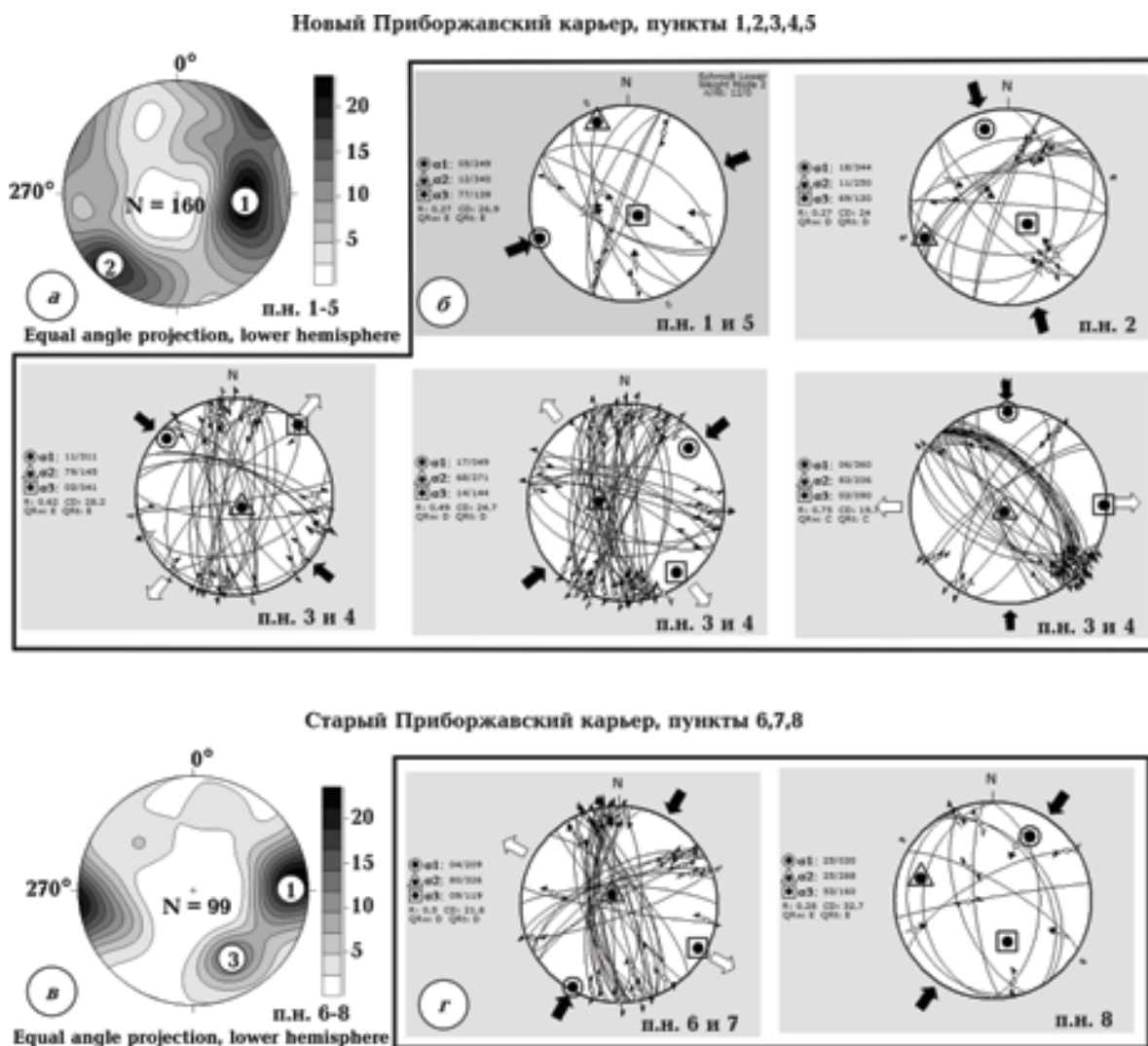
Рис. 5. Стереограммы для Приборжавских карьеров (нижняя полусфера, проекция Шмидта): а, в — изолинии концентрации полюсов тектонических зеркал (цифры в кружках — номера максимумов, описанных в тексте); б, г — кинематические стереограммы для групп тектонических зеркал (черные стрелки и кружки показывают ориентировку реконструированных осей сжатия, белые стрелки и квадраты — ориентировку осей растяжения).
