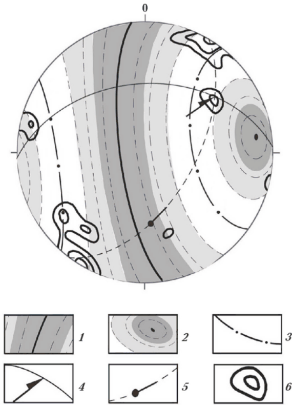
Рис. 2. Сегменты на стереограмме, в различной степени благоприятные для возникновения тектонических разрывов и вторичных смещений в пункте наблюдений Ordg_2 (здесь и далее — все построения на верхней полусфере): 1, 2 — проекция плоскости (1) и полюс (2) кальцитовой жилы, 3 — сечение \tau_{\max} , 4 — проекции плоскости зеркала скольжения и вектора смещения всяячего крыла, 5 — полюс зеркала и направление подвижки, 6 — изолинии плотности проекций векторов смещений (пояснения — в тексте).
