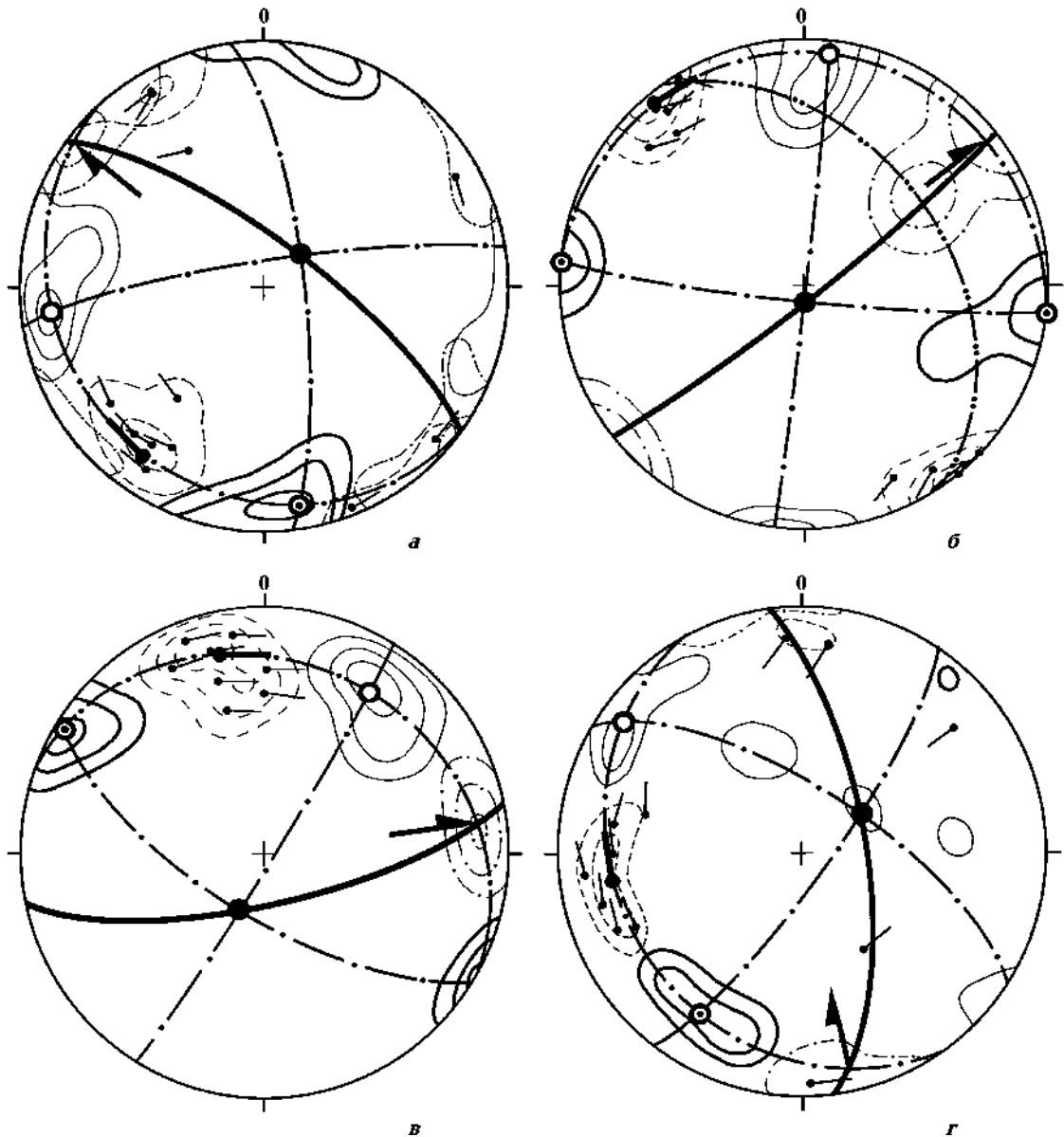
Рис. 7. Примеры СКП тектонических разрывов и смещений, сформированных в условиях сдвиговых деформационных режимов в обстановках субмеридионального сжатия (а), субмеридионального растяжения—субширотного сжатия (б), юго-восточного сжатия—северо-восточного растяжения (в), юго-западного сжатия—северо-западного растяжения (г). Условные обозначения см. на рис. 3.
