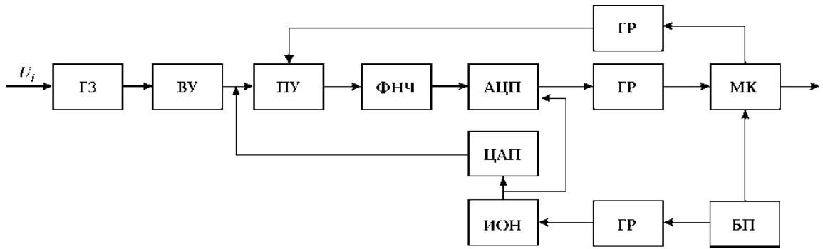
Рис. 3. Функциональная схема одного канала электрометра МТС LEMI-418: U_i — входное напряжение; ГЗ — схема защиты от грозовых разрядов и подачи большого напряжения на вход; ВУ — входной усилитель; ПУ — промежуточный усилитель с управляемым коэффициентом усиления; ФНЧ — фильтр нижних частот; АЦП — аналого-цифровой преобразователь; ЦАП — цифро-аналоговый преобразователь для компенсации начального смещения; ИОН — источник опорного напряжения; ГР — гальваническое разделение; МК — микроконтроллер для управления АЦП и ЦАП; БП — блок питания.
